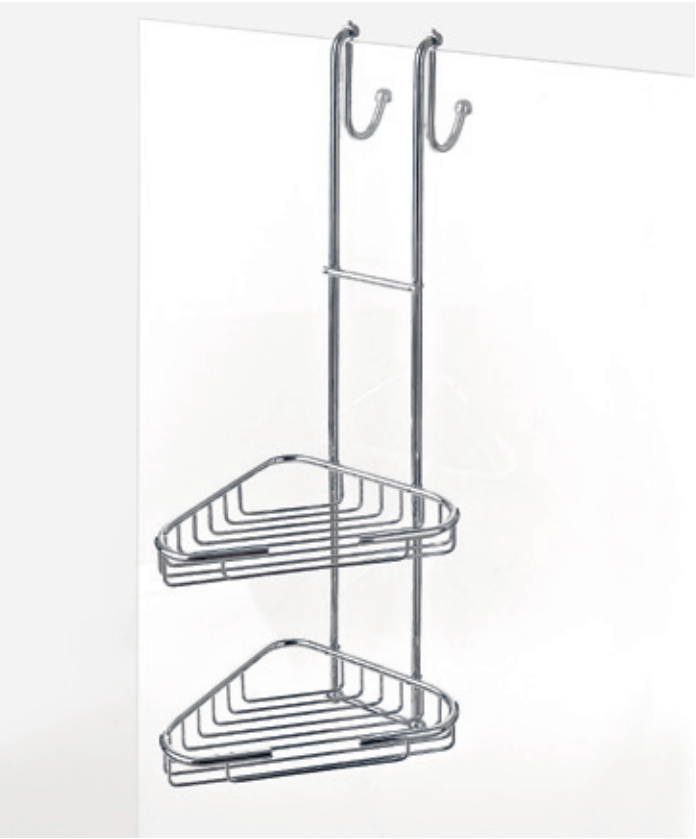
A202/R.4 Angolare doccia con gancio regolabile 2 piani per vetro filo lucido Double triangular shelf for shower with adjustable hook 24x28x68 cm LxPxH
